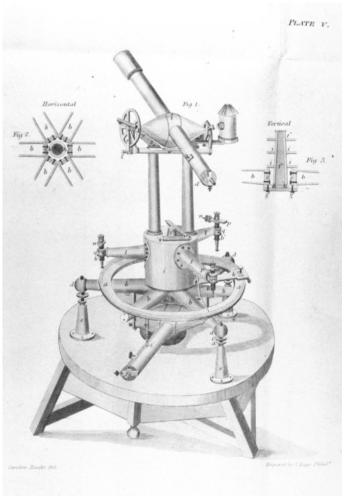
Illustration eines Troughton Theodoliten (ca. 70 cm). Caroline Hassler, 1820.
